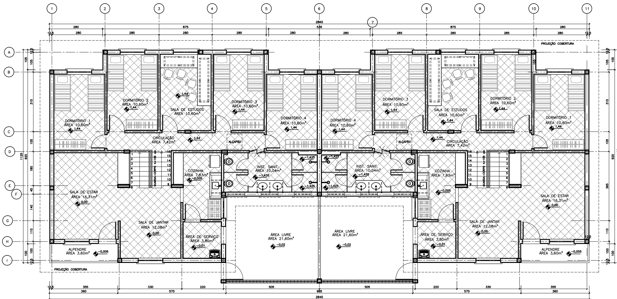
1 PLANTA LAYOUT TIPO 1 - TÉRREO E 1º PAVTO SEM ESCALA
