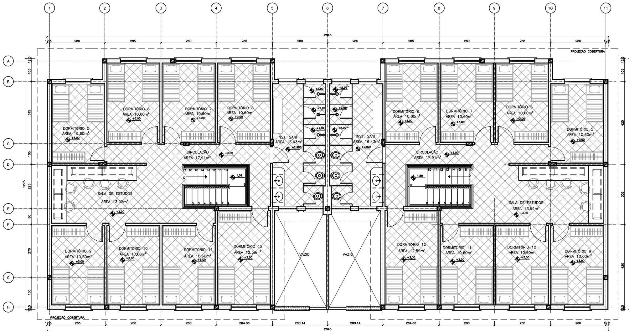
1 PLANTA BAIXA TIPO 2 - 1º PAVTO SEM ESCALA
