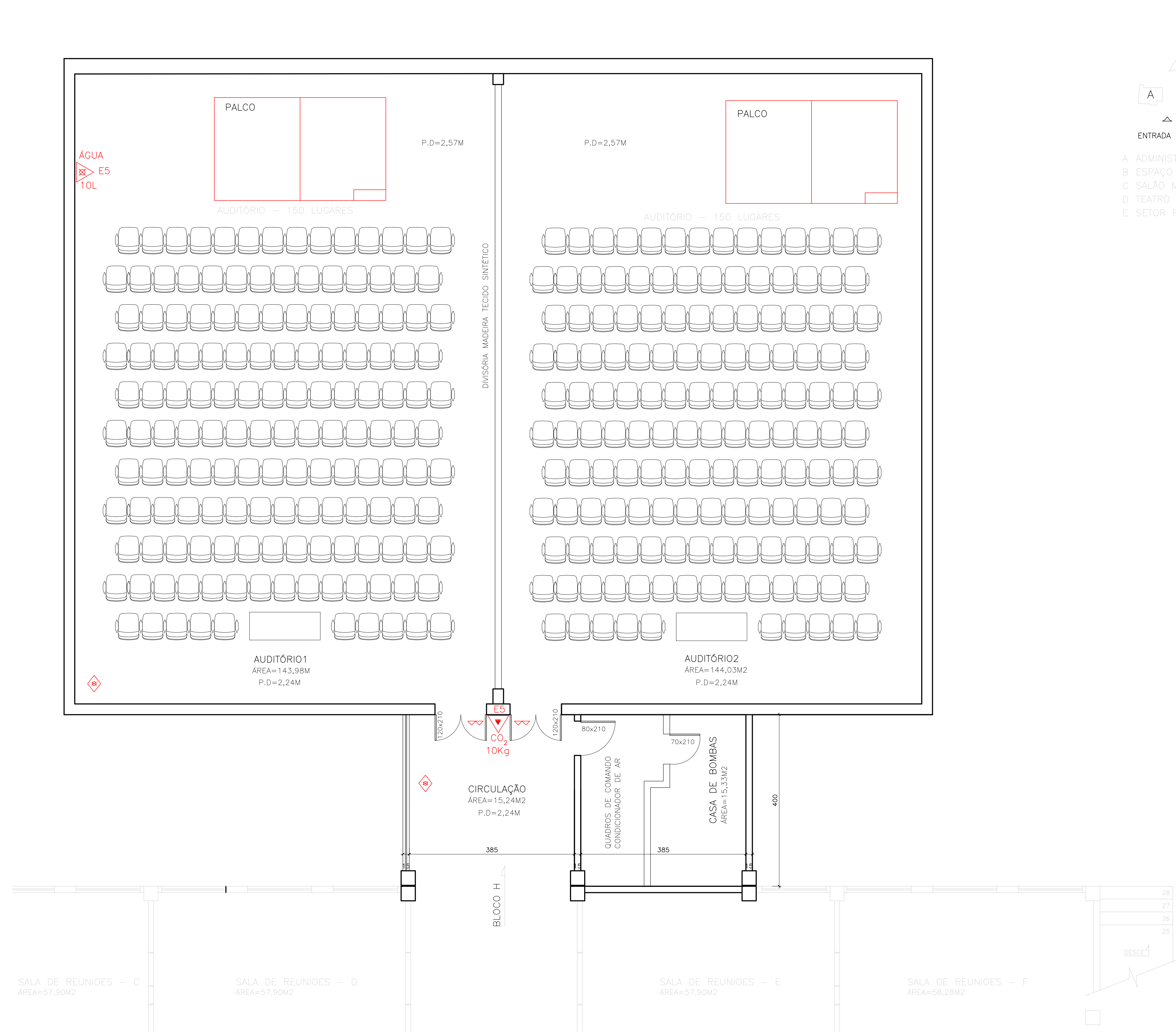
PLANTA BAIXA 2º PAVIMENTO – AUDITÓRIOS ESCALA 1:50 A=318,58M2
