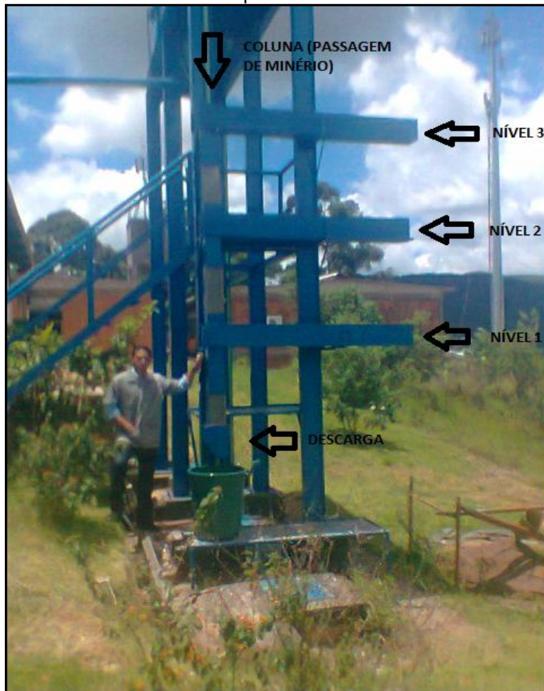
Vista frontal do modelo de passagem de minério, em trabalhos de bolsistas. (*)
