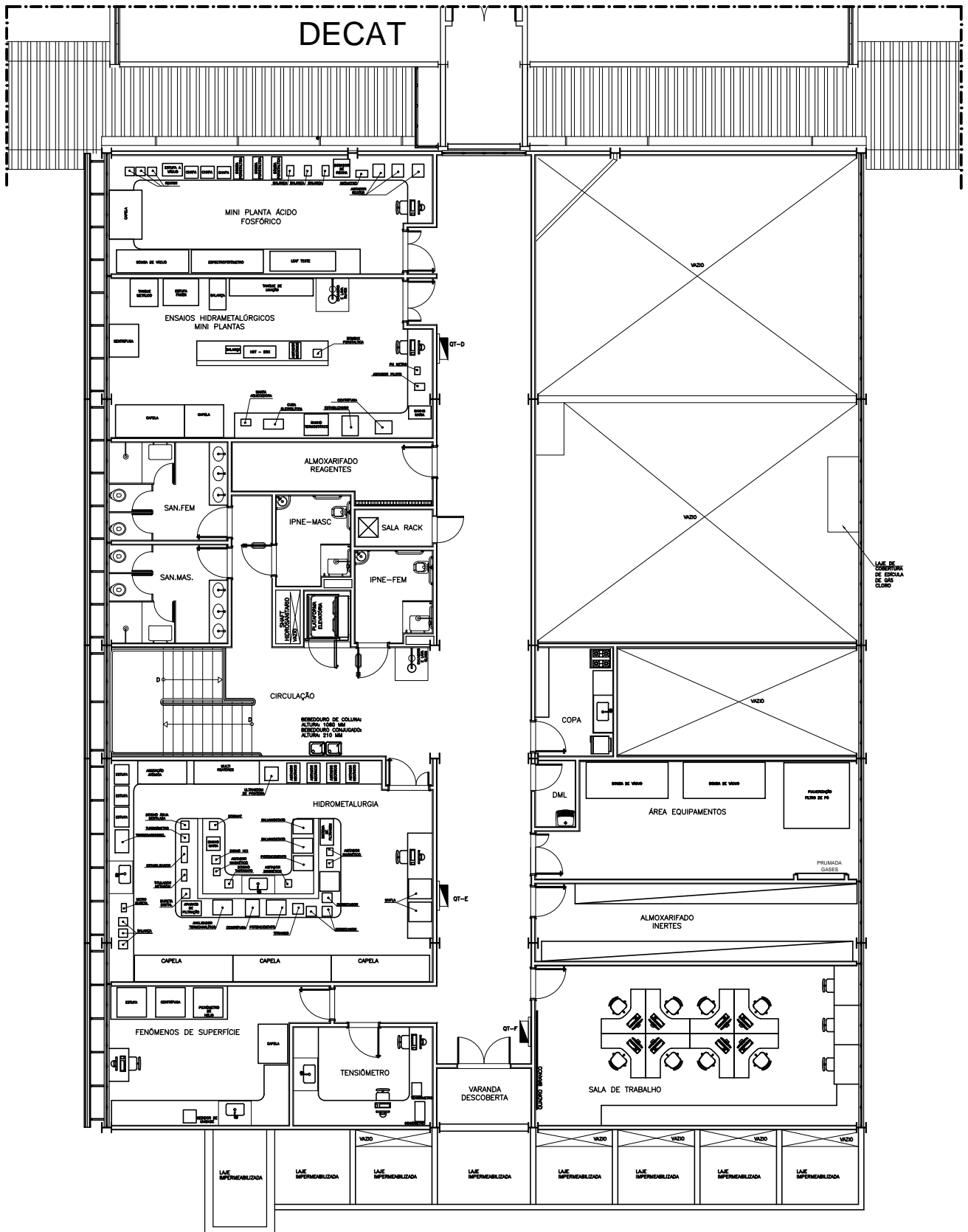
1 PLANTA LAYOUT - 1º PAVIMENTO SEM ESCALA
